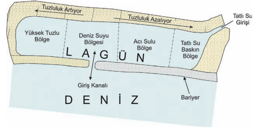
Tuz Gölü lagün suyu kütlesinin deniz ve akarsu su girişlerine göre tanımlanması
