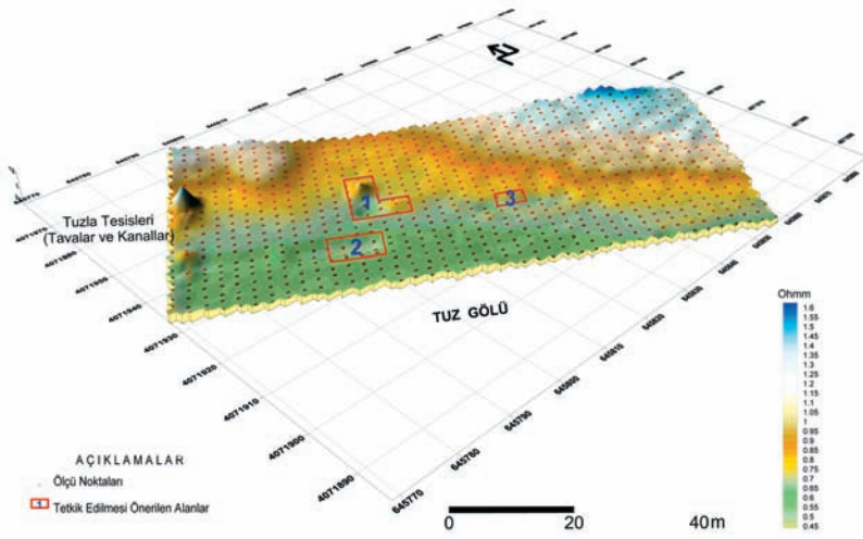
Tuzla'nın arkeojeofizik etüdü 3-B öz direnç anomali haritası
